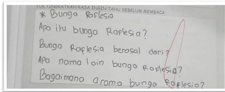
Gambar 2.7 Kolom Bertanya
