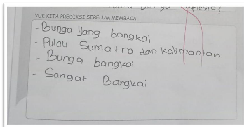
Gambar 2.8 Kolom Prediksi
