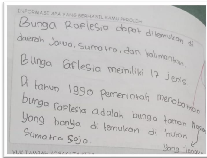
Gambar 2.9 Kolom Informasi
